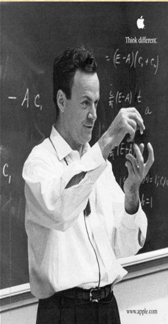
Feynmann
